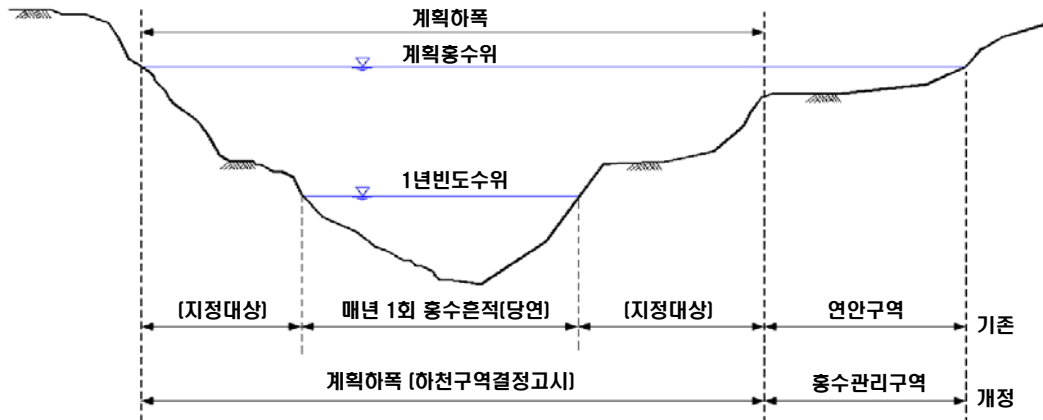
<그림-5> 하천구역의 설정방법-(3) 제방이 없는 곳
