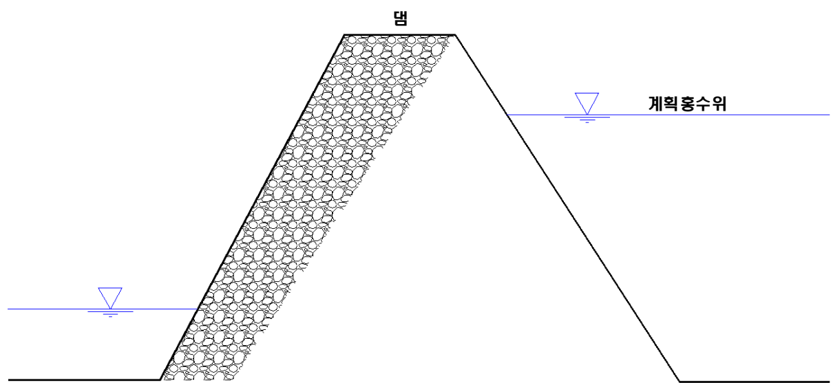
<그림-9> 하천구역의 설정방법-(7) 댐, 하구둑 등 저류시설
