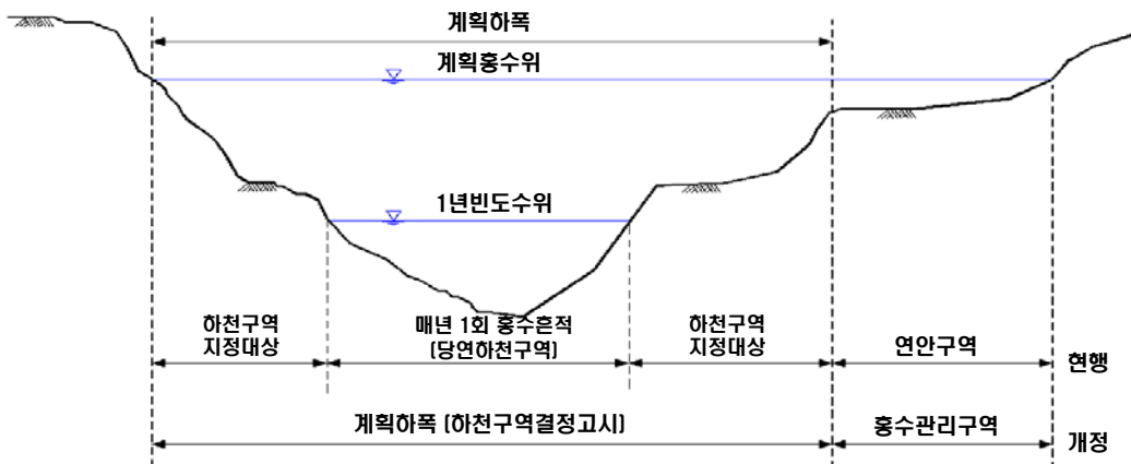
<그림-11> 홍수관리구역의 설정방법-(1) 하천기본계획 수립지역
