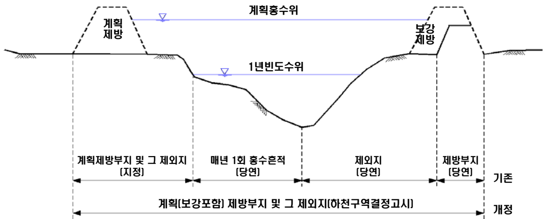
<그림-4> 하천구역의 설정방법-(2) 계획(보강)제방
