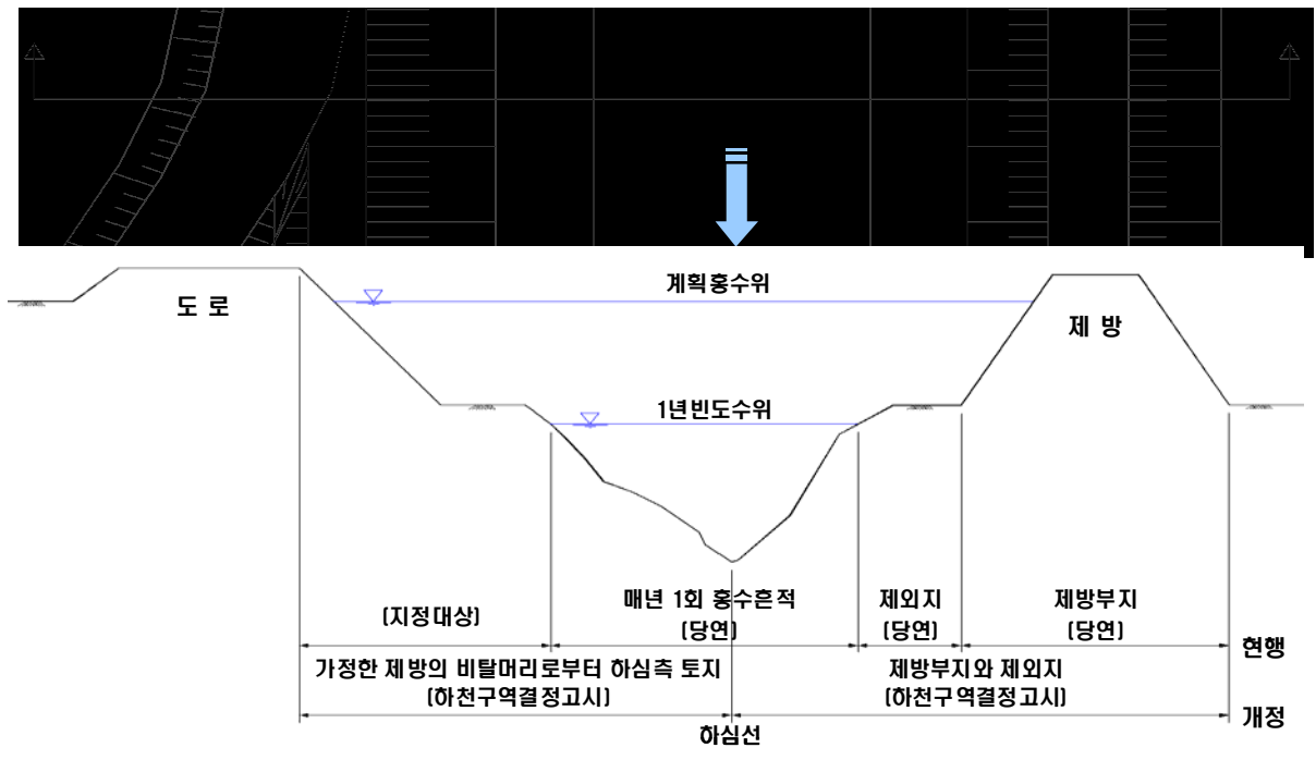
<그림-8> 하천구역의 설정방법-(6) 선형공작물이 제방의 역할을 하는 구간
