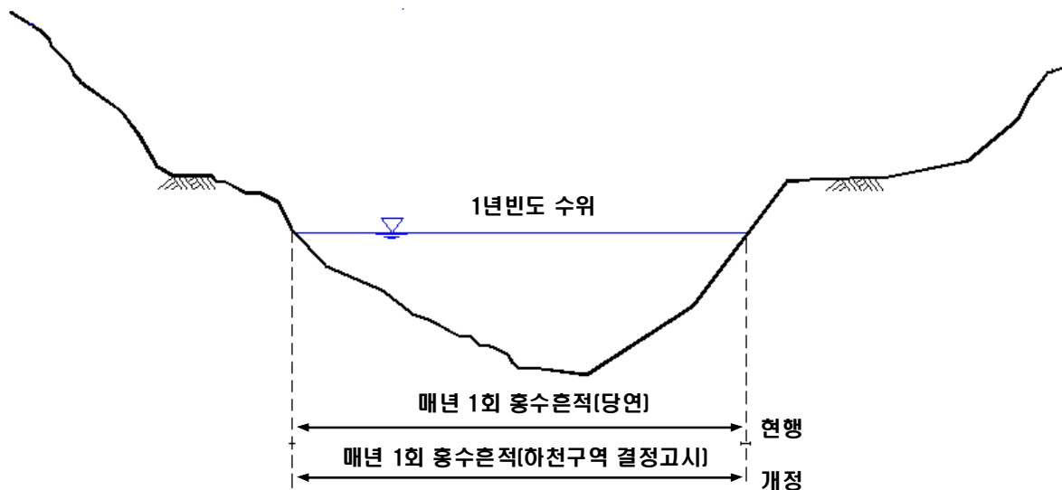
<그림-10> 하천구역의 설정방법-(8) 하천기본계획 미수립구간
