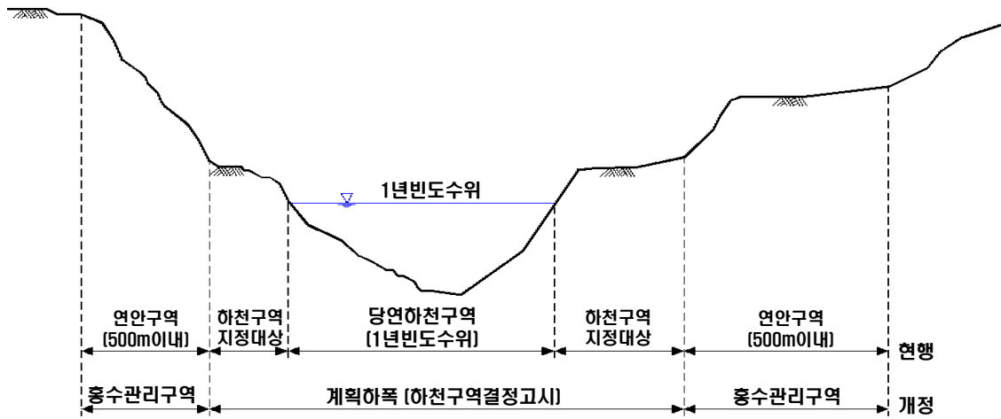
<그림-12> 홍수관리구역의 설정방법-(2) 하천기본계획 미수립 지역
