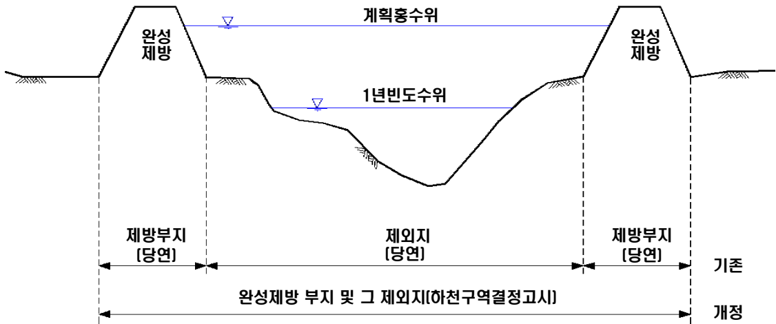
<그림-3> 하천구역의 설정방법-(1) 완성제방
