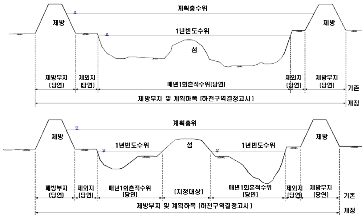
<그림-7> 하천구역의 설정방법-(5) 섬 형태(계획홍수위보다 낮은 곳)의 토지
