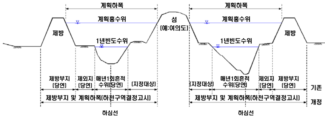
<그림-6> 하천구역의 설정방법-(4) 섬 형태(계획홍수위보다 높은 곳)의 토지
